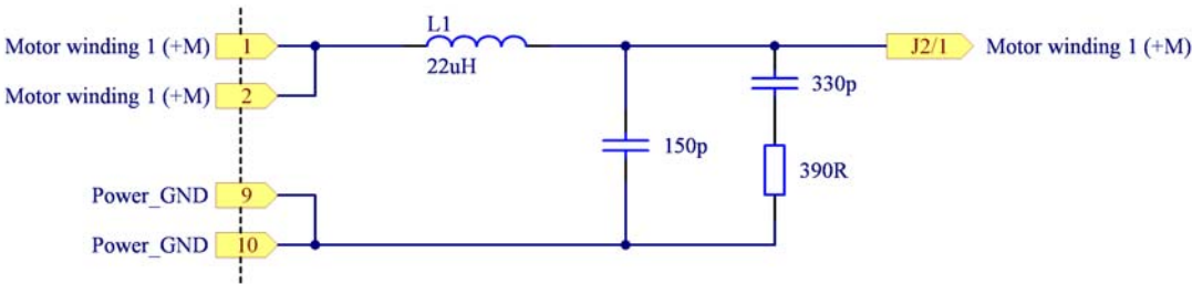
图 5-24 连接电机绕组 1（对于电机绕组 2 & 3 也类似）
