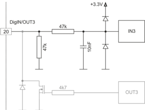
图 3-9 DigIN3 的连接（DigIN4 的连接方式类似）
