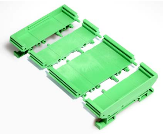
图 5-28 ESCON Module MoBo – 装到 DIN 导轨上
