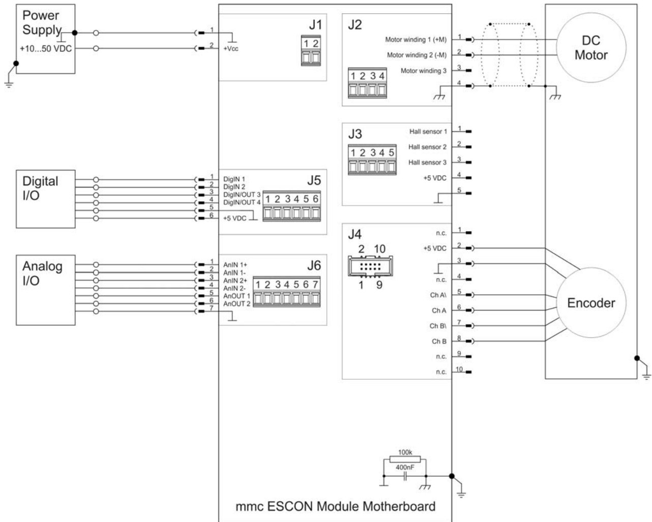
图 5-37 ESCON Module MoBo – 带编码器的 maxon DC motor (J2 / J4)
