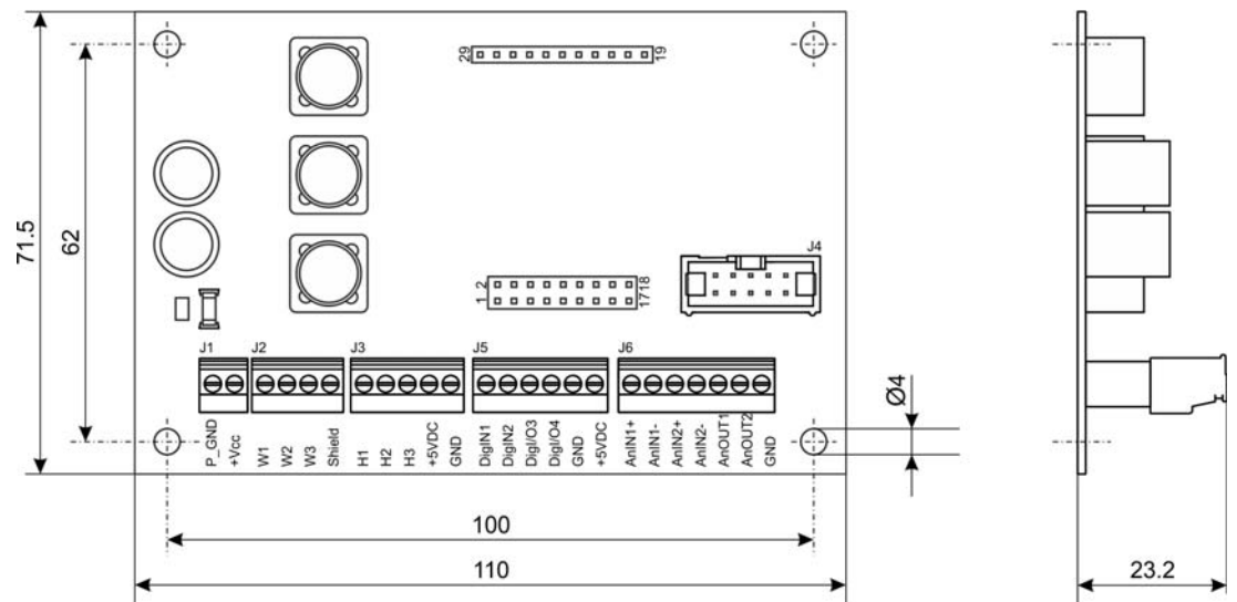
图 5-27 ESCON Module MoBo – 尺寸图 [mm]
