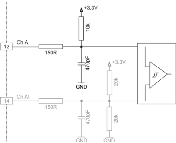
图 3-6 编码器输入端连接，通道 A 单端（通道 B 的连接方式类似）
