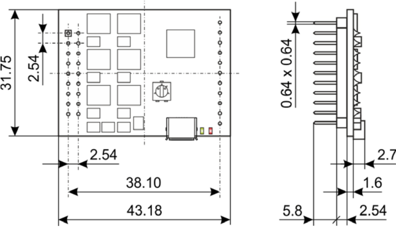
图 2-1 尺寸图 [mm]
