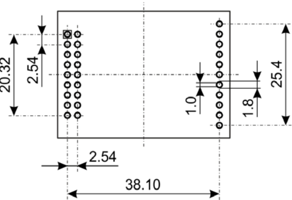
图 5-25 THT Footprint [mm] – 俯视图
