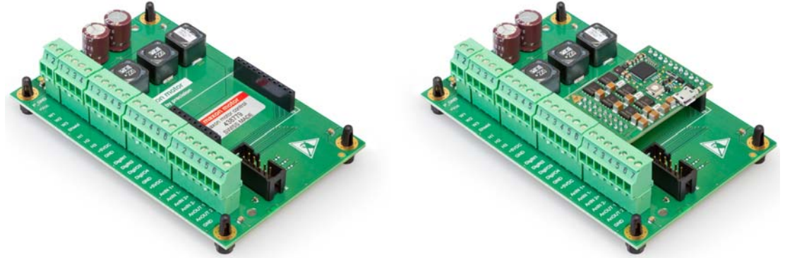
图 5-26 ESCON Module MoBo（左），其上是 ESCON Module 50/5（右）
