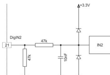
图 3-8 DigIN2 的连接
