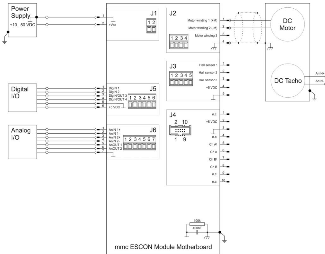
图 5-36 ESCON Module MoBo – 带直流测速发电机的 maxon DC motor (J2)
