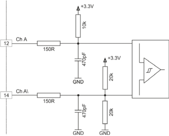
图 3-5 编码器输入端连接，通道 A 差分（通道 B 的连接方式类似）
