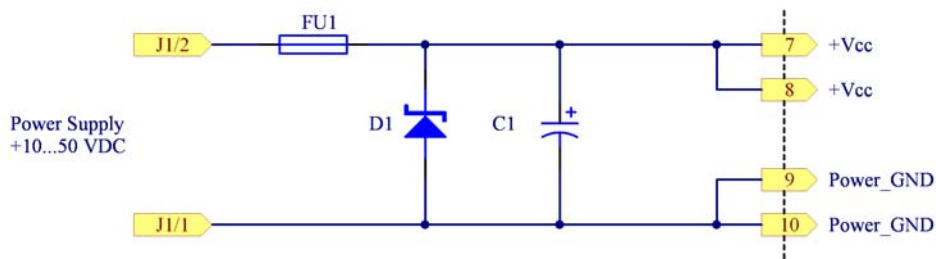
图 5-23 连接供电线路
