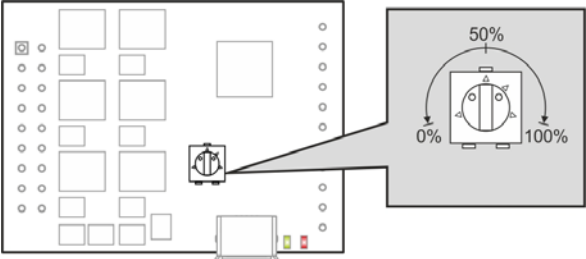
图 3-15 电位器 – 安装位置和调节范围
