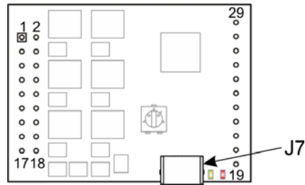
图 4-17 接口 – 名称和安装位置
