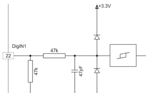
图 3-7 DigIN1 的连接
