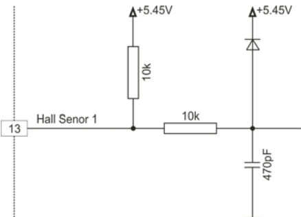
图 3-4 霍尔传感器 1 输入端的连接（霍尔传感器 2 和 3 的连接方式类似）
