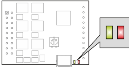
图 3-16 LED – 安装位置
