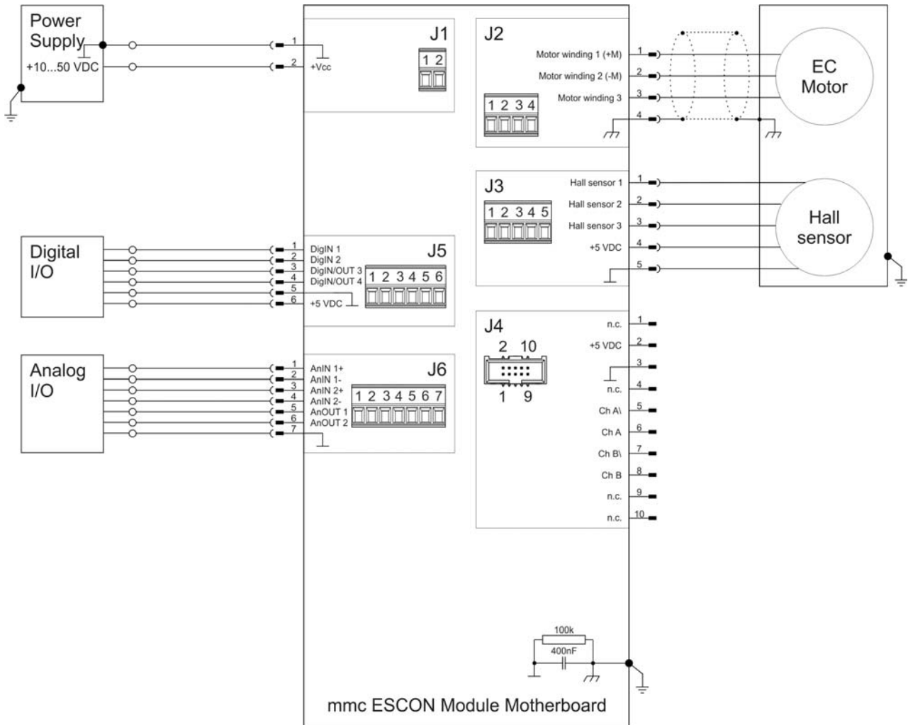
图 5-38 ESCON Module MoBo – 带霍尔传感器的 maxon EC motor (J2 / J3)
