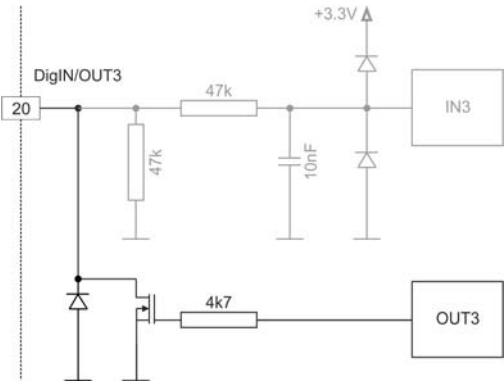
图 3-10 DigOUT3 的连接（DigOUT4 的连接方式类似）
