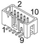
图 5-32 ESCON Module MoBo – 编码器接插件 J4
