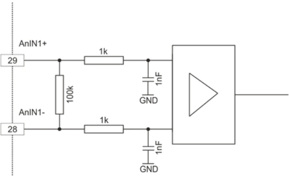
图 3-12 AnIN1 的连接（AnIN2 的连接方式类似）
