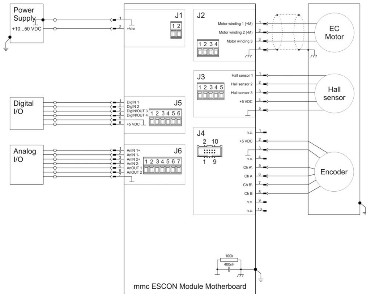
图 5-39 ESCON Module MoBo – 带霍尔传感器和编码器的 maxon EC motor (J2 / J3 / J4)
