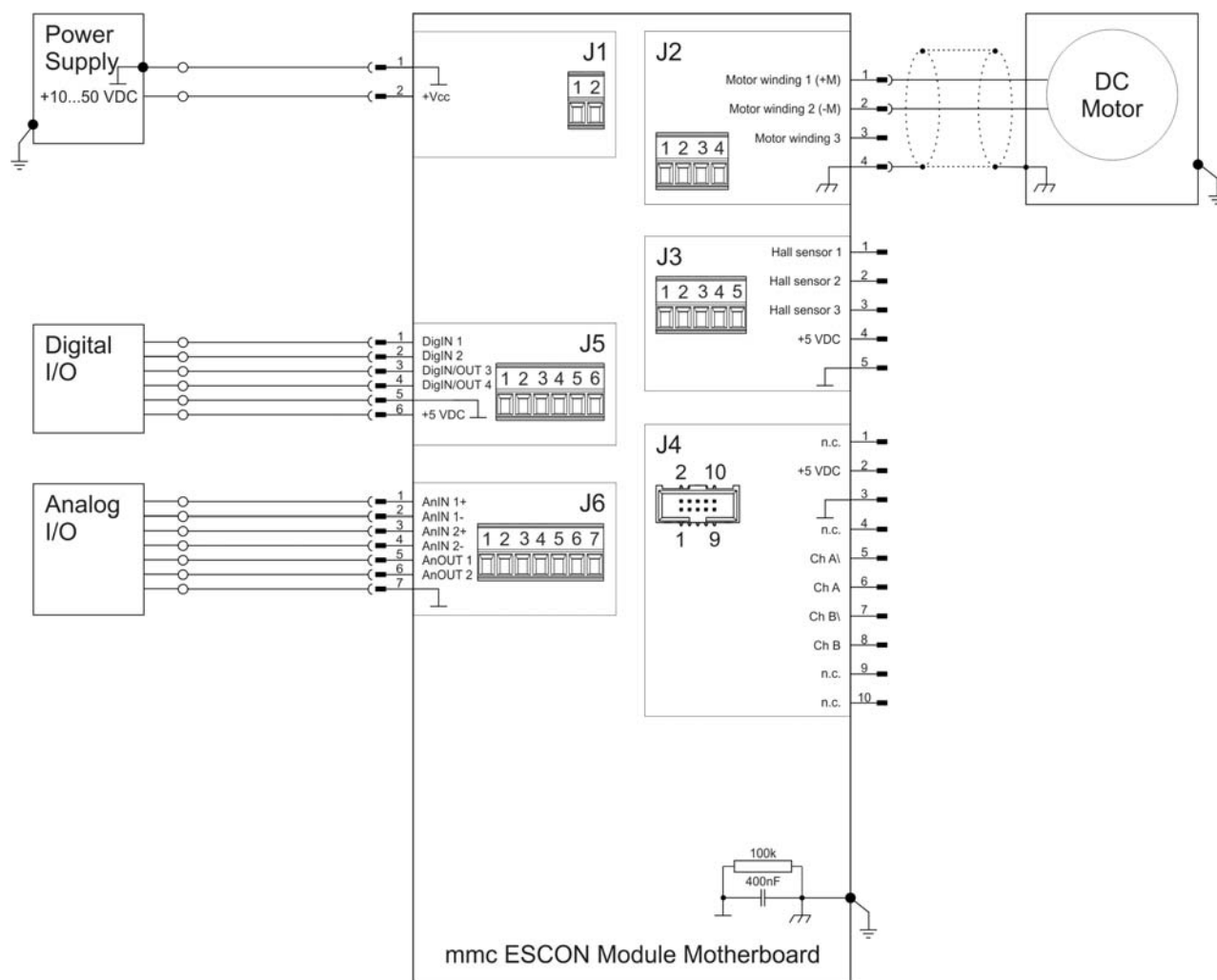
图 5-35 ESCON Module MoBo – maxon DC motor (J2)
