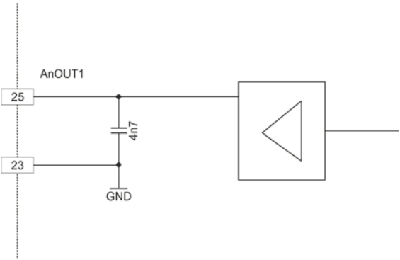
图 3-13 AnOUT1 的连接（AnOUT2 的连接方式类似）
